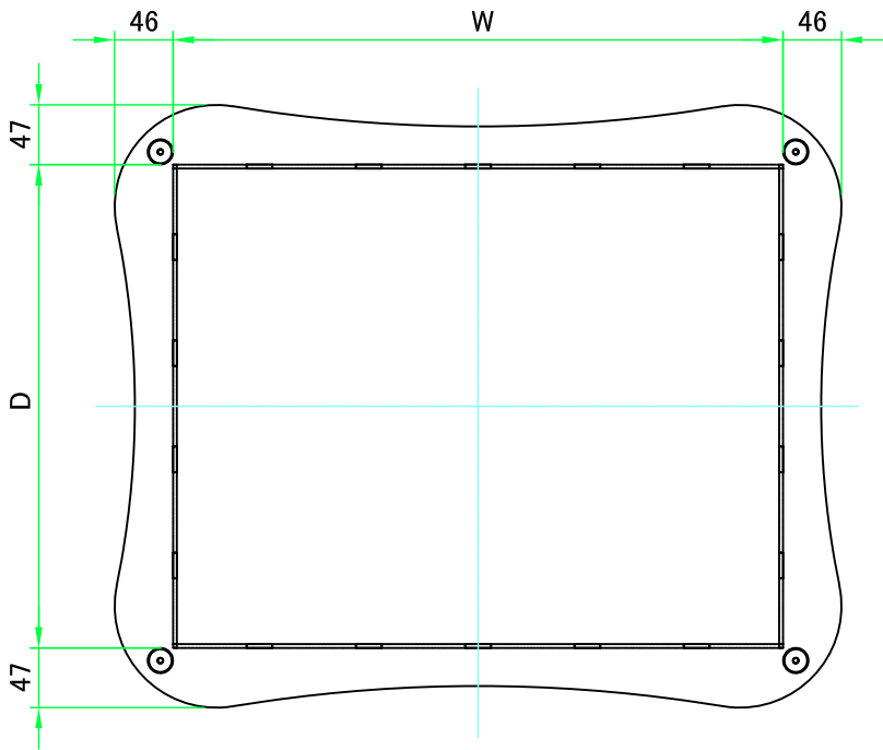
Wパネル1 / W panel 1
