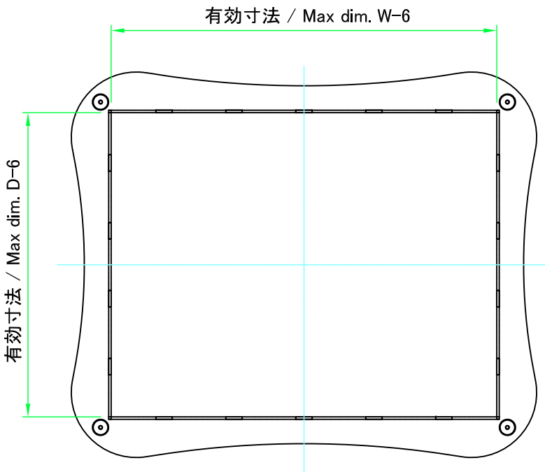
下カバー / Bottom cover
