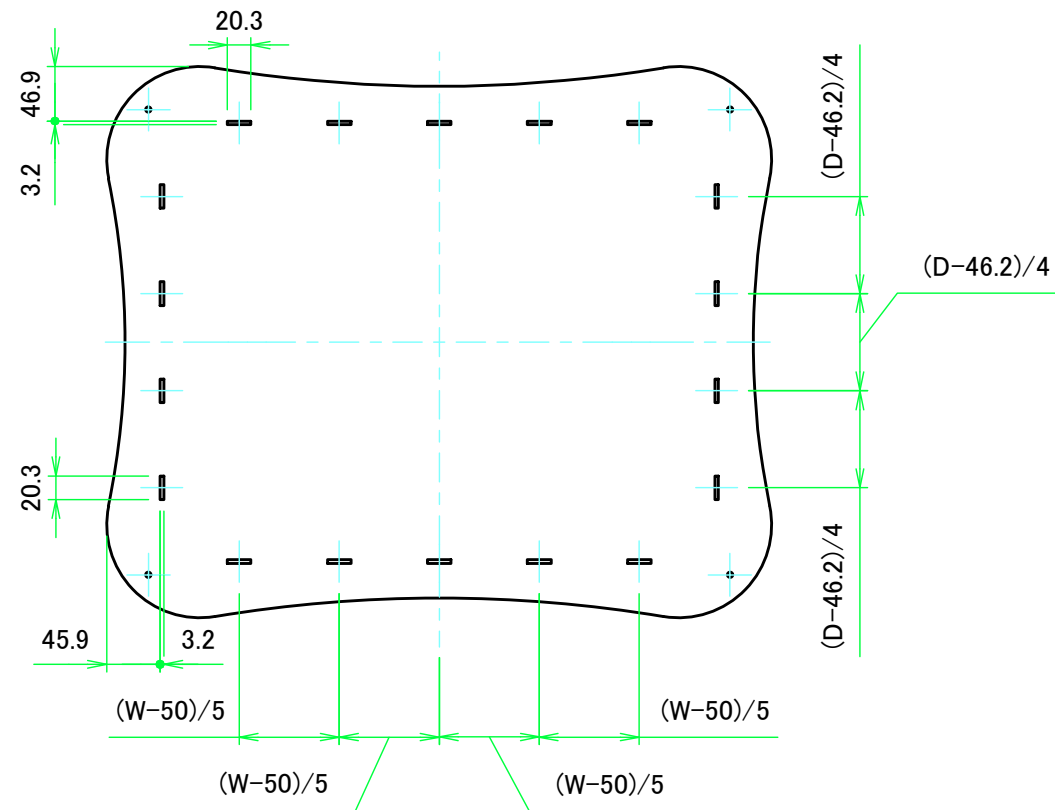
上カバー裏面 / Top cover Backside
